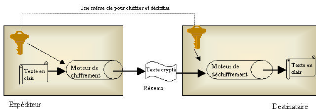
Figure 1: Schéma d'une transmission sécurisée par clé secrète.
